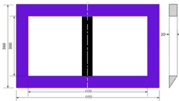
图 8 安全区围栏示意图
