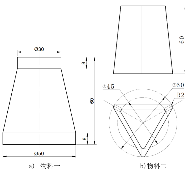
图 6 智能搬运赛项的物料形状与尺寸
