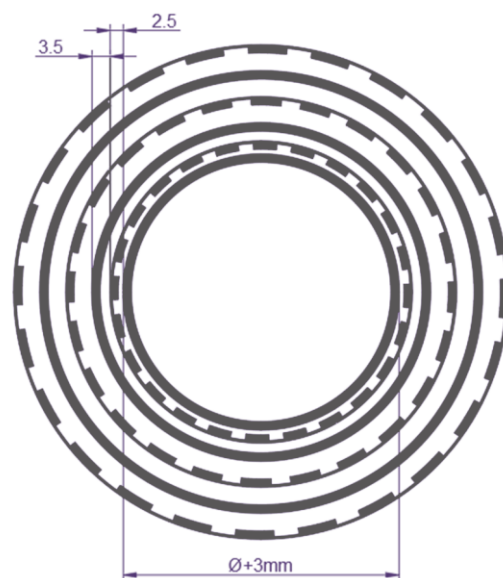
图 4 暂存区、粗加工区和精加工区的圆环
